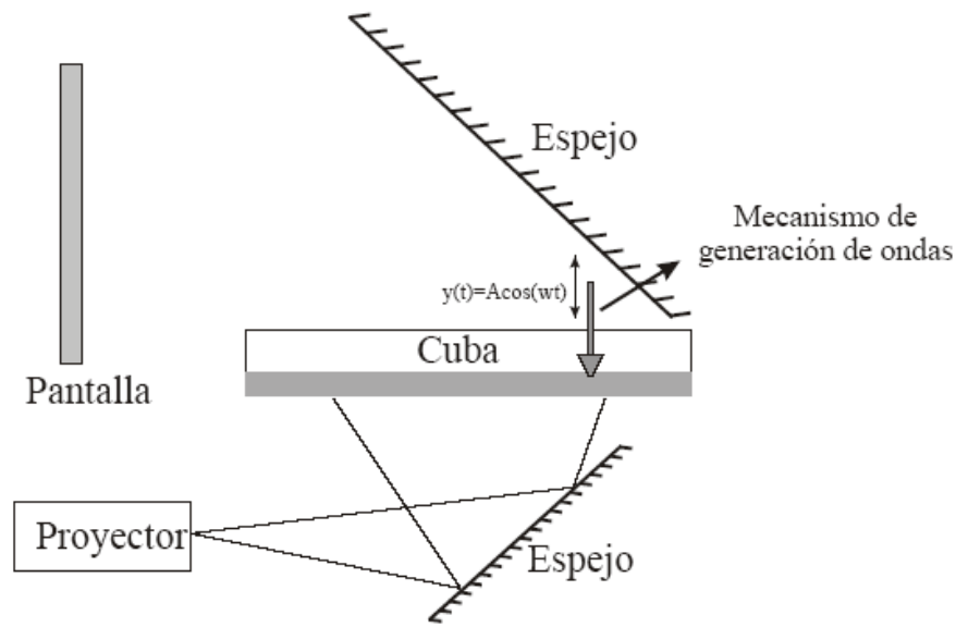
Figura. Montaje Experimental para Observar Interferencia de Ondas en Agua.
